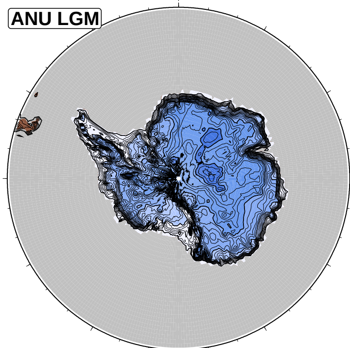
ANU LGM
